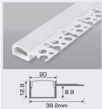
B20 - 1 T W39.2 x H12.9mm 1.5m 354.000 Nhôm định hình + Chụp nhựa Dẻo
