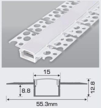
B15 - 2 T W55.3 x H12.8mm 1.5m 354.000 Nhôm định hình + Chụp nhựa Dẻo
