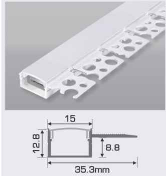
B15 - 1 T W35.3 x H12.8mm 1.5m 324.000 Nhôm định hình + Chụp nhựa Dẻo
