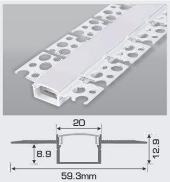
B20 - 2 T W59.3 x H12.9mm 1.5m 384.000 Nhôm định hình + Chụp nhựa Dẻo
