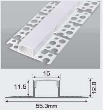
B15 - 2 D W55.3 x H12.8mm 1.5m 354.000 Nhôm định hình + Chụp nhựa Dẻo
